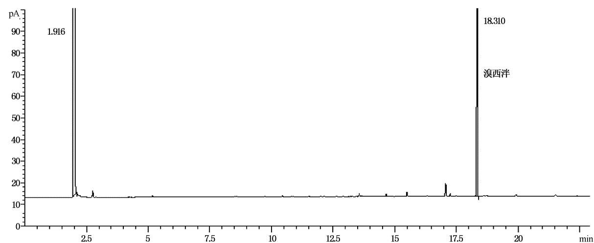
图 B.1 溴西洋气相色谱图
